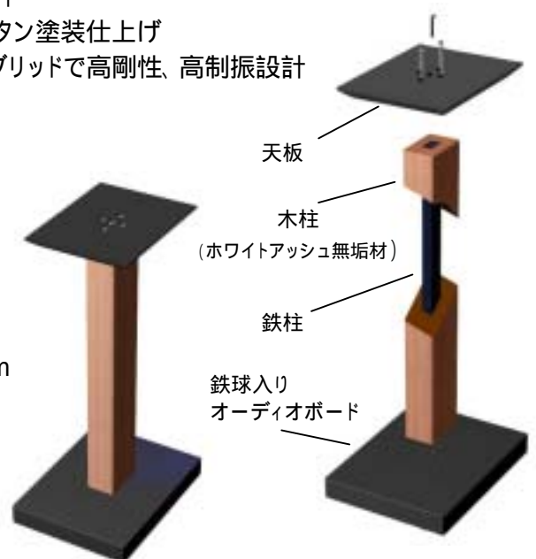
スピーカースタンド構成図
